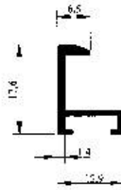
Profil No : 3110 Gramaj : 0.138 kg/m Çevre : 82 mm
