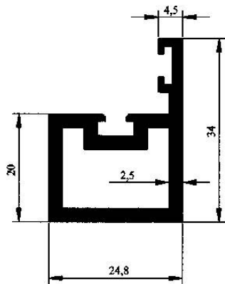
Profil No : 1903 Gramaj : 0.713 kg/m Çevre : 145 mm
