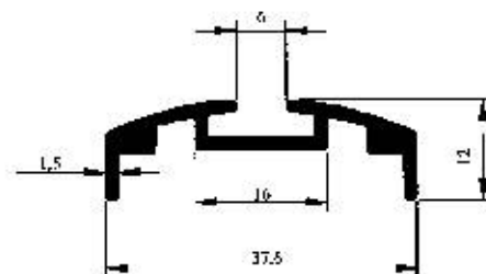
Profil No : 2611 Gramaj : 0.331 kg/m Çevre : 137 mm
