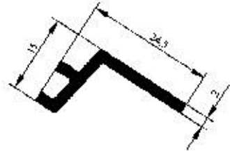
Profil No : 2320 Gramaj : 0.213 kg/m Çevre : 81 mm
