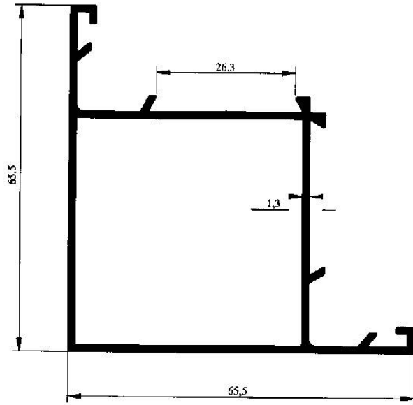
Profil No : 2027 Gramaj : 0.892 kg/m Çevre : 322 mm
