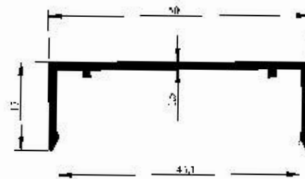
Profil No : 4015 Gramaj : 0.341 kg/m Çevre : 170 mm
