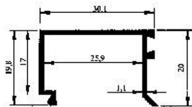
Profil No : 3636 Gramaj : 0.234 kg/m Çevre : 153 mm
