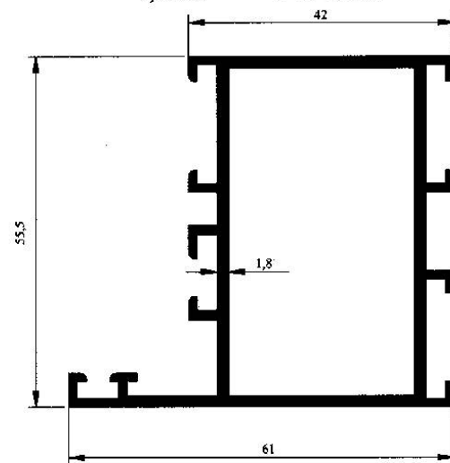
Profil No : 2529 Gramaj : 1.173 kg/m Çevre : 357 mm
