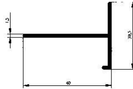
Profil No : 2319 Gramaj : 1.198 kg/m Çevre : 206 mm
