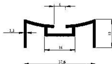
Profil No : 2612 Gramaj : 0.331 kg/m Çevre : 163 mm
