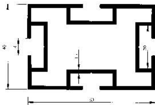
Profil No : 3148 Gramaj : 1.391 kg/m Çevre : 357 mm
