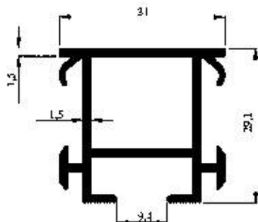
Profil No : 2463 Gramaj : 0.588 kg/m Çevre : 223 mm
