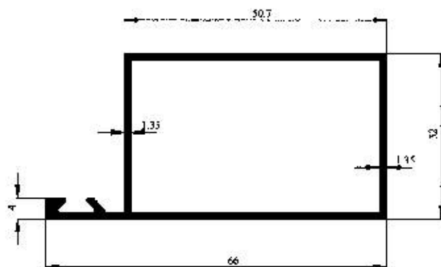
Profil No : 2616 Gramaj : 0.678 kg/m Çevre : 208 mm
