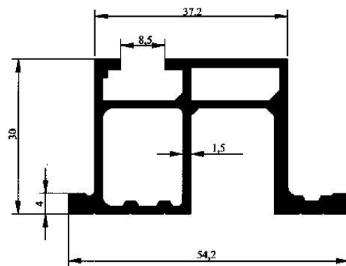
Profil No : 2796 Gramaj : 0.926 kg/m Çevre : 241 mm
