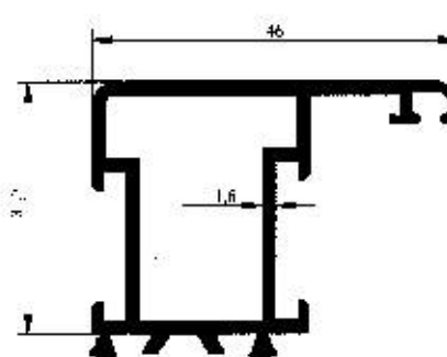
Profil No : 2335 Gramaj : 0.722 kg/m Çevre : 237 mm
