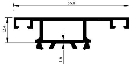
Profil No : 2544 Gramaj : 0.564 kg/m Çevre : 216 mm
