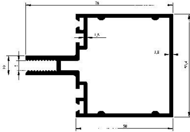
Profil No : 3557 Gramaj : 1.474 kg/m Çevre : 347 mm
