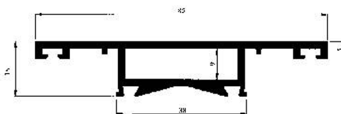
Profil No : 2368 Gramaj : 0.972 kg/m Çevre : 236 mm
