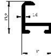
Profil No : 3162 Gramaj : 0.179 kg/m Çevre : 84 mm
