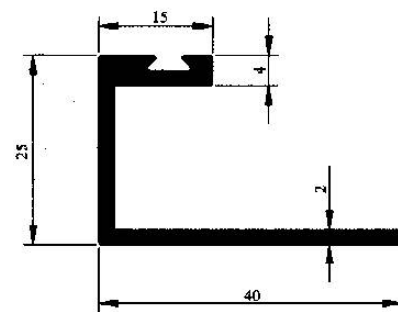
Profil No : 2602 Gramaj : 0.547 kg/m Çevre : 183 mm
