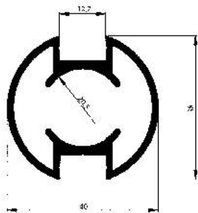
Profil No : 4716 Gramaj : 0.851 kg/m Çevre : 152 mm
