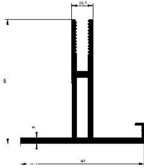
Profil No : 2243 Gramaj : 1.315 kg/m Çevre : 316 mm
