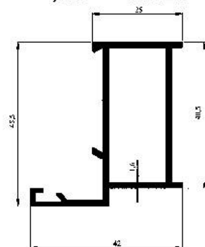
Profil No : 2152 Gramaj : 0.812 kg/m Çevre : 278 mm
