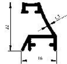
Profil No : 3165 Gramaj : 0.236 kg/m Çevre : 127 mm
