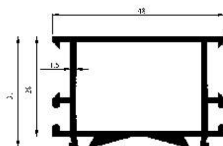
Profil No : 2369 Gramaj : 0.799 kg/m Çevre : 238 mm
