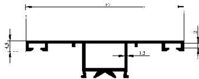
Profil No : 2414 Gramaj : 0.296 kg/m Çevre : 169 mm
