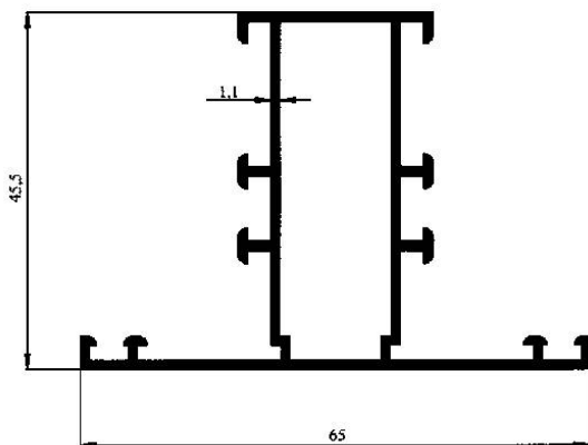
Profil No : 2520 Gramaj : 0.699 kg/m Çevre : 343 mm
