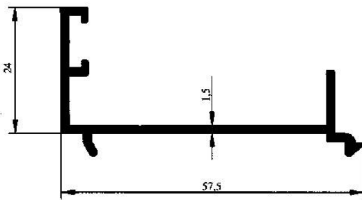
Profil No : 1963 Gramaj : 0.442 kg/m Çevre : 219 mm
