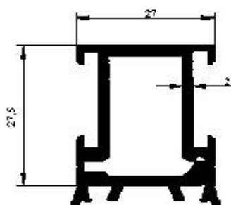
Profil No : 2316 Gramaj : 0.688 kg/m Çevre : 180 mm
