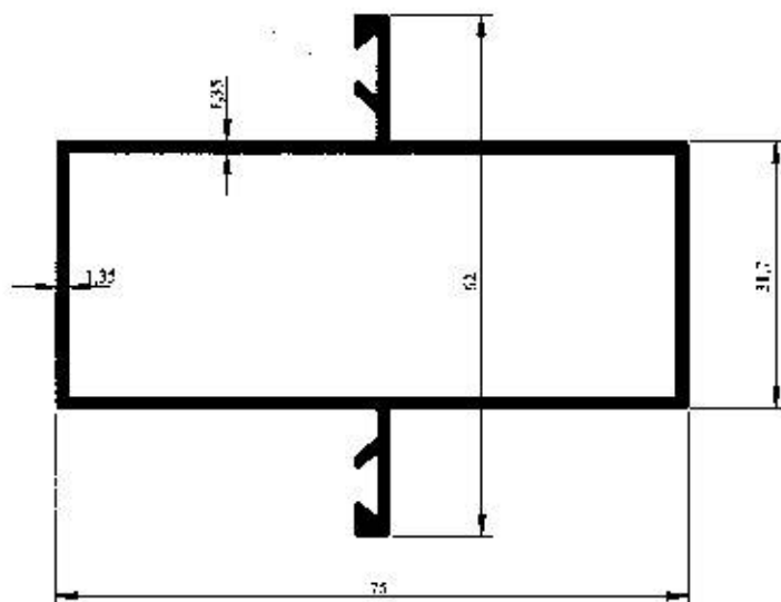
Profil No : 2614 Gramaj : 0.943 kg/m Çevre : 298 mm
