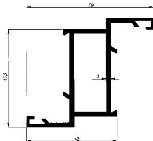
Profil No : 2151 Gramaj : 0.963 kg/m Çevre : 278 mm
