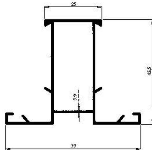
Profil No : 2124 Gramaj : 0.515 kg/m Çevre : 285 mm
