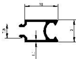
Profil No : 3783 Gramaj : 0.195 kg/m Çevre : 116 mm
