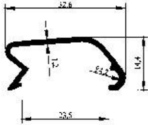
Profil No : 2733 Gramaj : 0.195 kg/m Çevre : 119 mm
