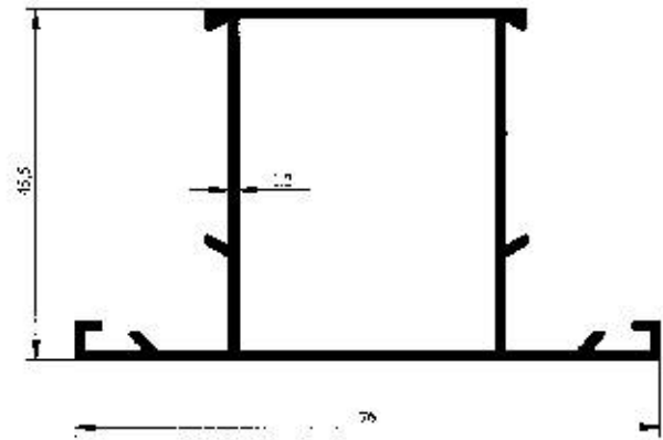
Profil No : 2038 Gramaj : 0.766 kg/m Çevre : 304 mm
