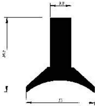
Profil No : 2227 Gramaj : 1.046 kg/m Çevre : 125 mm
