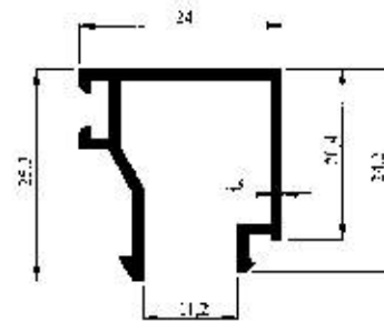
Profil No : 2414 Gramaj : 0.296 kg/m Çevre : 169 mm
