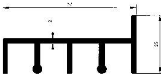
Profil No : 1959 Gramaj : 0.761 kg/m Çevre : 268 mm
