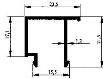
Profil No : 1964 Gramaj : 0.229 kg/m Çevre : 140 mm
