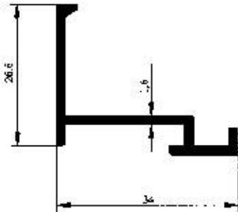
Profil No : 2300 Gramaj : 0.318 kg/m Çevre : 148 mm
