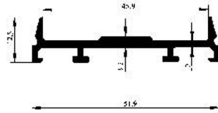
Profil No : 2787 Gramaj : 0.470 kg/m Çevre : 177 mm
