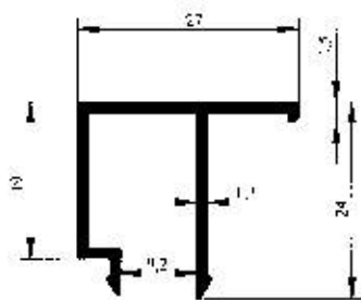
Profil No : 2440 Gramaj : 0.525 kg/m Çevre : 210 mm
