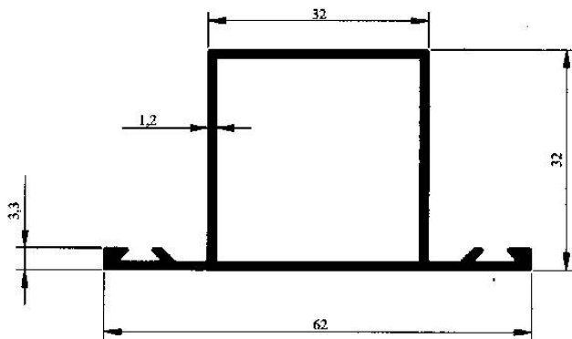
Profil No : 2603 Gramaj : 0.569 kg/m Çevre : 206 mm
