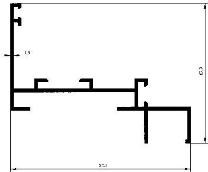
Profil No : 4018 Gramaj : 0.919 kg/m Çevre : 445 mm
