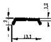
Profil No : 3880 Gramaj : 0.048 kg/m Çevre : 32 mm
