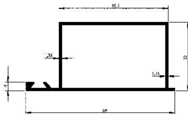
Profil No : 2617 Gramaj : 0.688 kg/m Çevre : 214 mm
