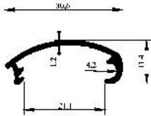
Profil No : 2766 Gramaj : 0.170 kg/m Çevre : 100 mm
