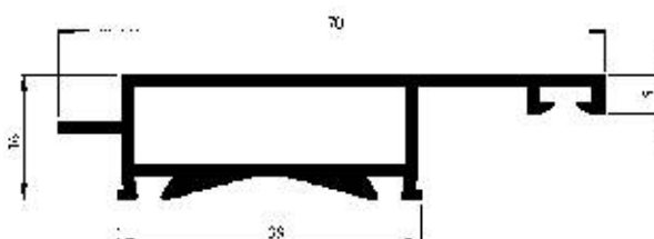
Profil No : 2375 Gramaj : 0.680 kg/m Çevre : 213 mm
