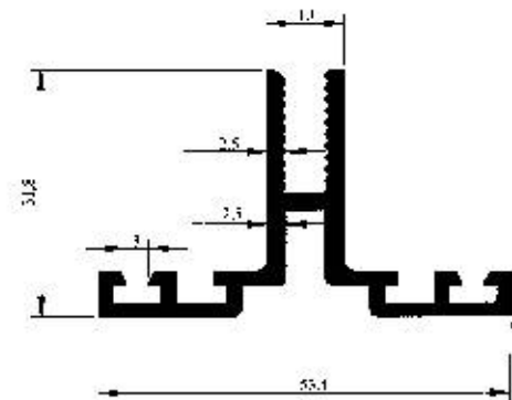
Profil No : 3556 Gramaj : 0.756 kg/m Çevre : 284 mm
