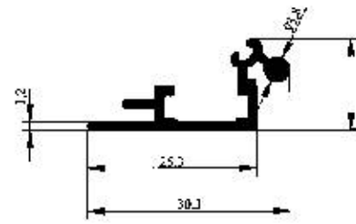
Profil No : 2757 Gramaj : 0.227 kg/m Çevre : 126 mm
