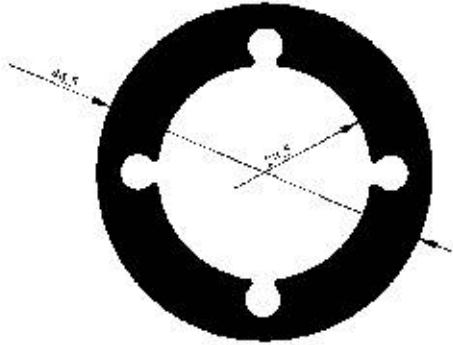
Profil No : 2225 Gramaj : 2.278 kg/m Çevre : 140 mm
