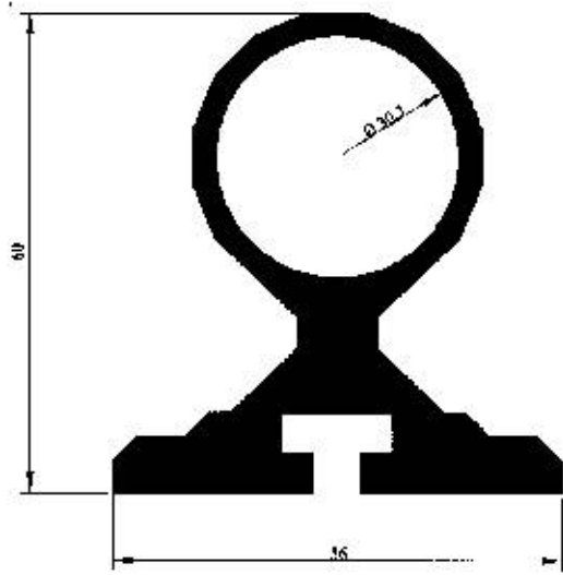
Profil No : 3854 Gramaj : 2.217 kg/m Çevre : 229 mm
