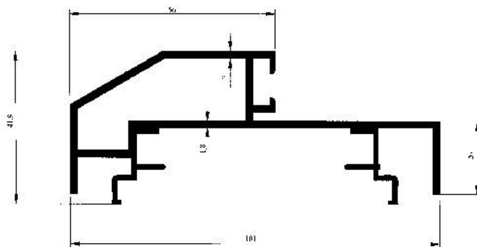
Profil No : 4096 Gramaj : 1.499 kg/m Çevre : 473 mm
