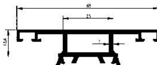
Profil No : 2315 Gramaj : 0.714 kg/m Çevre : 244 mm
