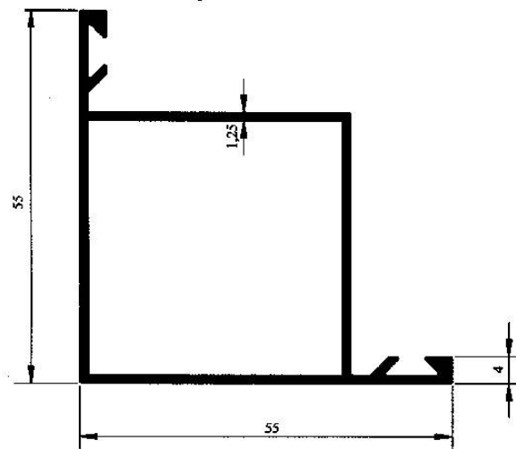
Profil No : 2623 Gramaj : 0.699 kg/m Çevre : 247 mm
