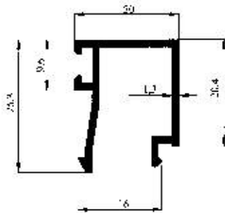
Profil No : 2415 Gramaj : 0.280 kg/m Çevre : 160 mm
