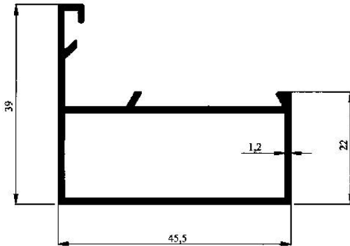
Profil No : 2084 Gramaj : 0.209 kg/m Çevre : 151 mm
