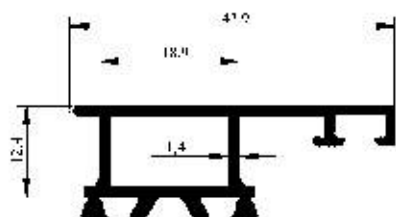
Profil No : 2347 Gramaj : 0.483 kg/m Çevre : 197 mm
