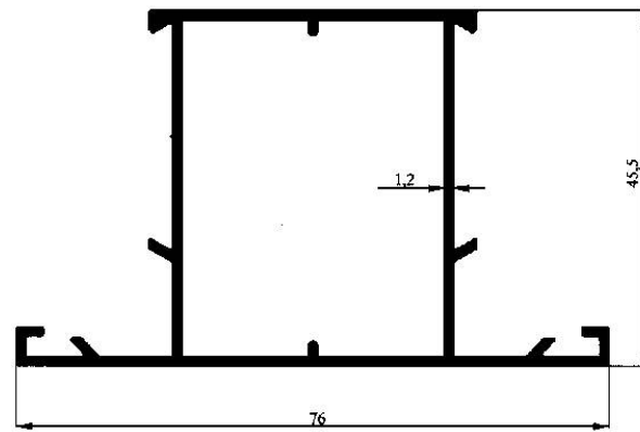
Profil No : 2174 Gramaj : 0.778 kg/m Çevre : 304 mm
