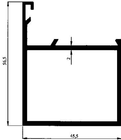
Profil No : 2173 Gramaj : 0.998 kg/m Çevre : 233 mm
