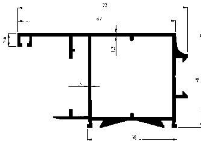
Profil No : 2452 Gramaj : 0.930 kg/m Çevre : 334 mm
