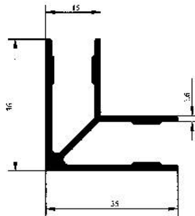
Profil No : 4489 Gramaj : 0.640 kg/m Çevre : 257 mm
