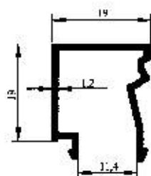
Profil No : 2332 Gramaj : 0.231 kg/m Çevre : 141 mm
