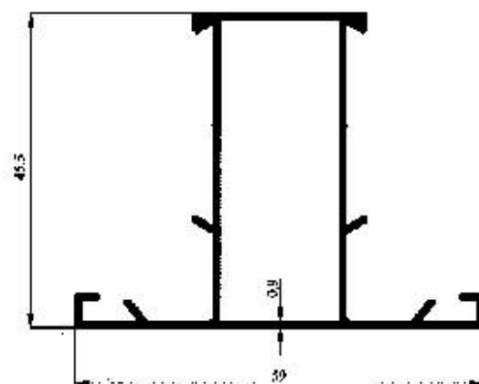
Profil No : 2128 Gramaj : 0.522 kg/m Çevre : 273 mm
