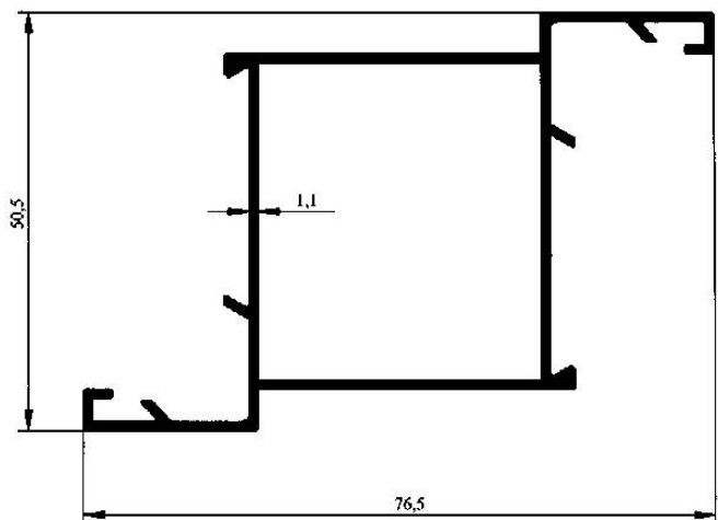
Profil No : 2020 Gramaj : 0.712 kg/m Çevre : 315 mm
