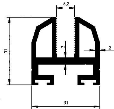
Profil No : 1902 Gramaj : 0.904 kg/m Çevre : 231 mm
