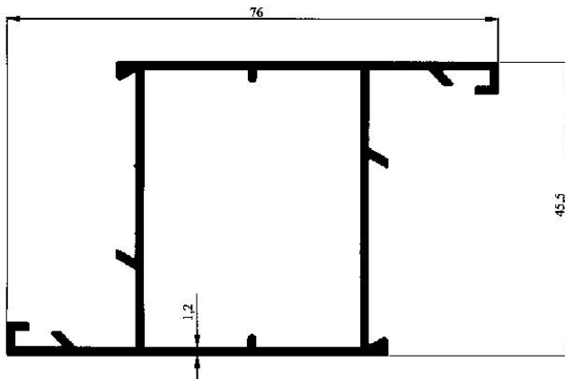
Profil No : 2173 Gramaj : 0.998 kg/m Çevre : 233 mm
