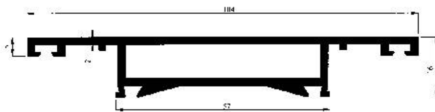
Profil No : 2452 Gramaj : 0.930 kg/m Çevre : 334 mm
