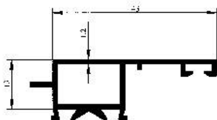
Profil No : 2444 Gramaj : 0.390 kg/m Çevre : 174 mm
