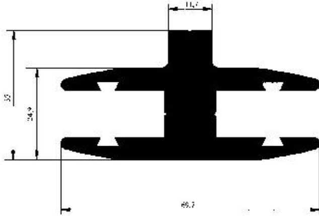
Profil No : 2239 Gramaj : 2.715 kg/m Çevre : 333 mm
