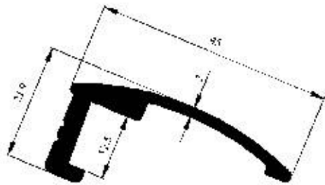
Profil No : 3030 Gramaj : 0.527 kg/m Çevre : 133 mm
