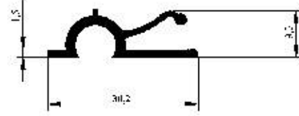
Profil No : 2897 Gramaj : 0.245 kg/m Çevre : 115 mm
