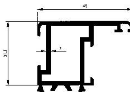
Profil No : 2315 Gramaj : 0.714 kg/m Çevre : 244 mm
