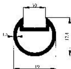
Profil No : 4728 Gramaj : 0.257 kg/m Çevre : 68 mm
