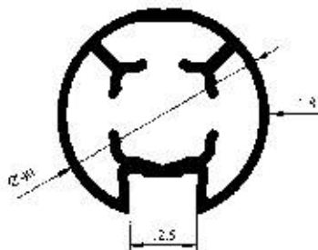
Profil No : 3032 Gramaj : 0.940 kg/m Çevre : 142 mm
