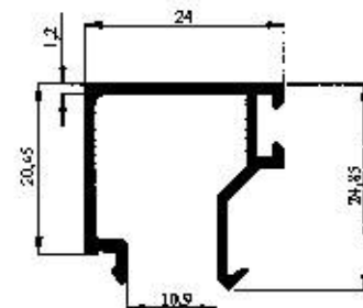
Profil No : 2496 Gramaj : 0.280 kg/m Çevre : 168 mm
