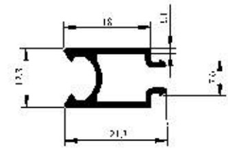
Profil No : 2665 Gramaj : 0.196 kg/m Çevre : 119 mm
