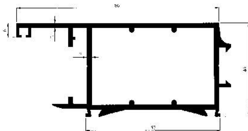
Profil No : 2455 Gramaj : 1.178 kg/m Çevre : 301 mm
