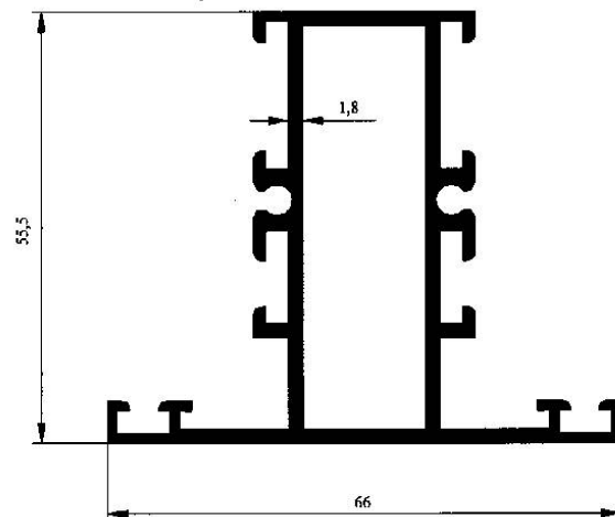
Profil No : 2527 Gramaj : 1.241 kg/m Çevre : 404 mm
