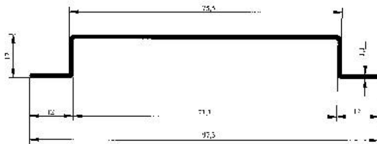
Profil No : 3867 Gramaj : 0.352 kg/m Çevre : 236 mm
