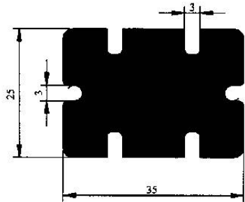
Profil No : 2252 Gramaj : 1.854 kg/m Çevre : 225 mm
