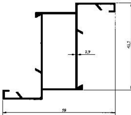
Profil No : 2125 Gramaj : 0.515 kg/m Çevre : 285 mm
