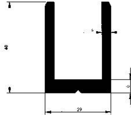
Profil No : 2319 Gramaj : 1.198 kg/m Çevre : 206 mm
