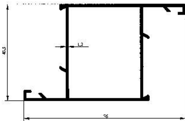
Profil No : 2039 Gramaj : 0.766 kg/m Çevre : 304 mm
