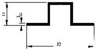
Profil No : 2794 Gramaj : 0.154 kg/m Çevre : 106 mm
