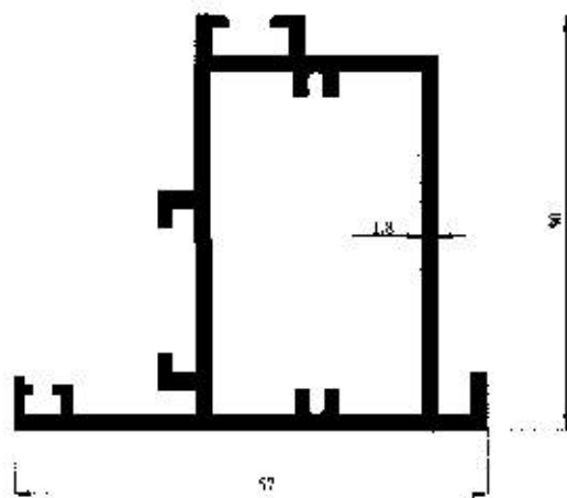
Profil No : 2439 Gramaj : 1.069 kg/m Çevre : 291 mm
