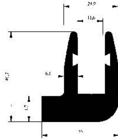
Profil No : 2245 Gramaj : 1.854 kg/m Çevre : 209 mm
