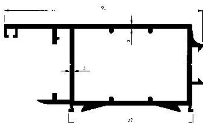
Profil No : 2373 Gramaj : 1.509 kg/m Çevre : 368 mm
