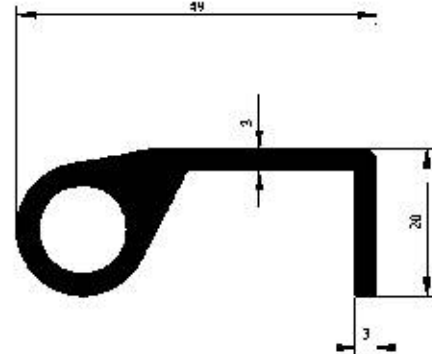
Profil No : 3856 Gramaj : 0.916 kg/m Çevre : 154 mm
