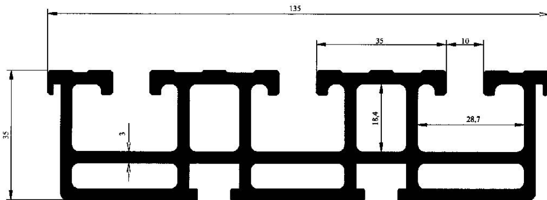
Profil No : 2252 Gramaj : 1.854 kg/m Çevre : 225 mm
