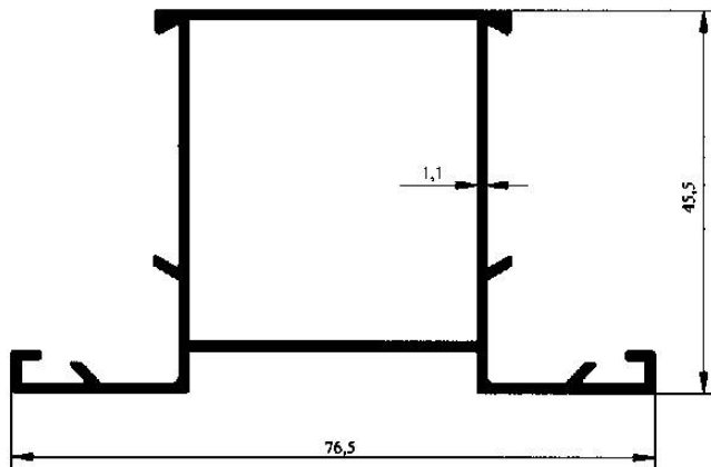
Profil No : 2019 Gramaj : 0.712 kg/m Çevre : 315 mm
