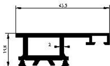
Profil No : 2316 Gramaj : 0.688 kg/m Çevre : 180 mm
