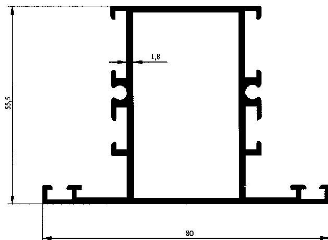
Profil No : 2528 Gramaj : 1.374 kg/m Çevre : 588 mm
