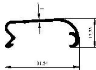
Profil No : 2799 Gramaj : 0.166 kg/m Çevre : 114 mm
