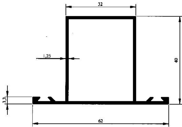
Profil No : 2601 Gramaj : 0.623 kg/m Çevre : 222 mm
