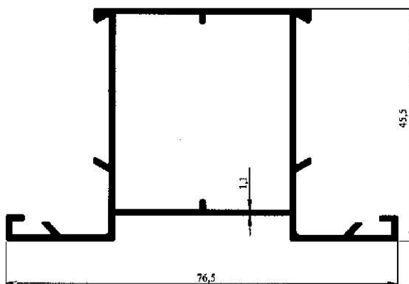
Profil No : 2177 Gramaj : 0.723 kg/m Çevre : 315 mm
