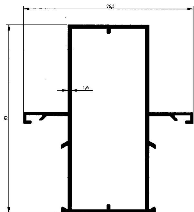
Profil No : 2020 Gramaj : 0.712 kg/m Çevre : 315 mm
