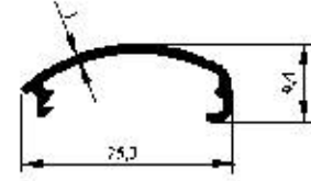
Profil No : 2741 Gramaj : 0.106 kg/m Çevre : 78 mm
