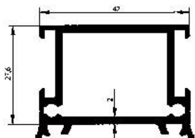
Profil No : 2312 Gramaj : 0.851 kg/m Çevre : 210 mm
