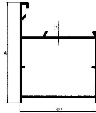
Profil No : 2174 Gramaj : 0.778 kg/m Çevre : 304 mm
