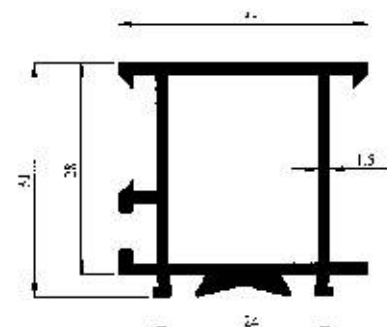
Profil No : 2468 Gramaj : 0.621 kg/m Çevre : 191 mm
