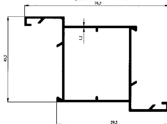
Profil No : 2176 Gramaj : 0.672 kg/m Çevre : 245 mm
