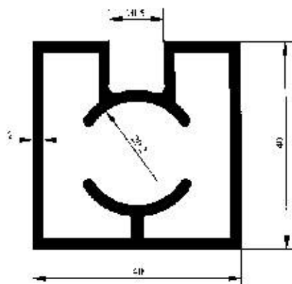
Profil No : 4725 Gramaj : 1.153 kg/m Çevre : 178 mm
