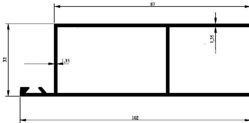
Profil No : 2618 Gramaj : 0.940 kg/m Çevre : 352 mm
