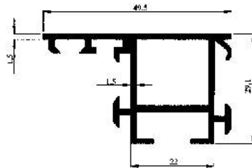
Profil No : 2462 Gramaj : 0.718 kg/m Çevre : 279 mm
