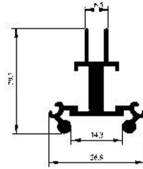
Profil No : 2934 Gramaj : 0.429 kg/m Çevre : 189 mm
