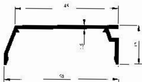
Profil No : 4014 Gramaj : 0.333 kg/m Çevre : 166 mm
