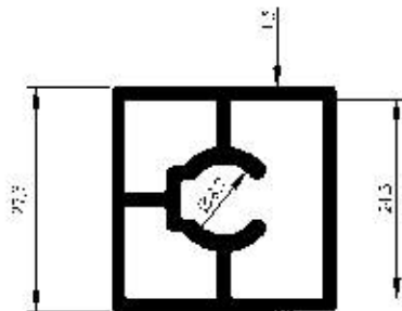
Profil No : 1937 Gramaj : 0.636 kg/m Çevre : 108 mm
