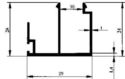
Profil No : 2944 Gramaj : 0.296 kg/m Çevre : 195 mm
