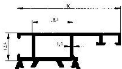
Profil No : 2347 Gramaj : 0.483 kg/m Çevre : 197 mm
