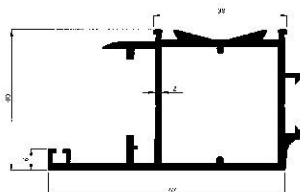
Profil No : 2372 Gramaj : 1.289 kg/m Çevre : 330 mm
