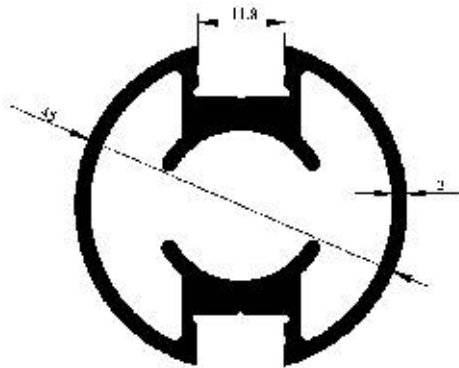
Profil No : 2256 Gramaj : 0.212 kg/m Çevre : 43 mm
