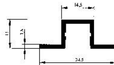
Profil No : 3866 Gramaj : 0.269 kg/m Çevre : 118 mm
