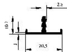
Profil No : 3177 Gramaj : 0.119 kg/m Çevre : 70 mm
