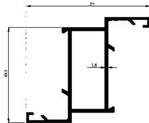
Profil No : 2150 Gramaj : 0.812 kg/m Çevre : 278 mm
