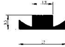
Profil No : 2245 Gramaj : 1.854 kg/m Çevre : 209 mm
