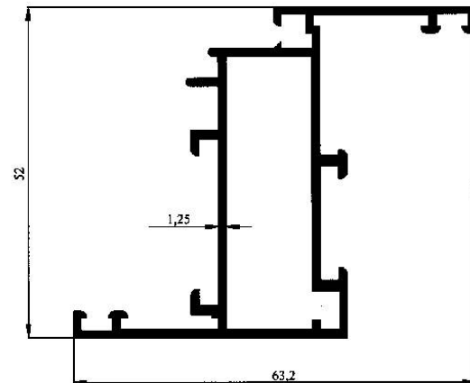
Profil No : 2519 Gramaj : 0.789 kg/m Çevre : 349 mm
