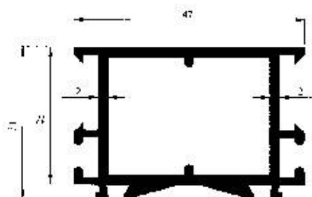
Profil No : 2368 Gramaj : 0.972 kg/m Çevre : 236 mm
