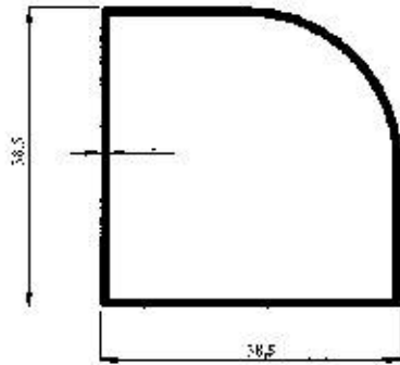
Profil No : 2135 Gramaj : 0.384 kg/m Çevre : 145 mm
