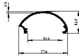
Profil No : 2797 Gramaj : 0.116 kg/m Çevre : 92 mm
