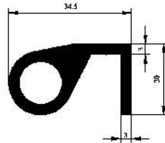
Profil No : 3857 Gramaj : 0.800 kg/m Çevre : 125 mm
