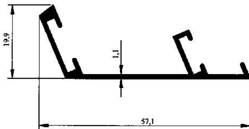
Profil No : 2793 Gramaj : 0.332 kg/m Çevre : 201 mm
