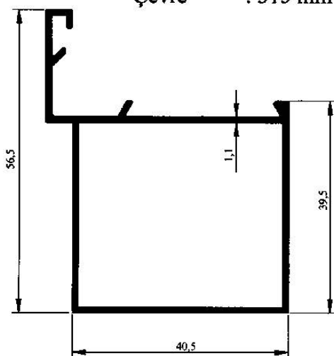
Profil No : 2019 Gramaj : 0.712 kg/m Çevre : 315 mm
