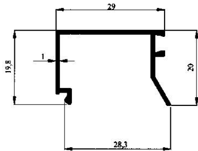
Profil No : 2084 Gramaj : 0.209 kg/m Çevre : 151 mm
