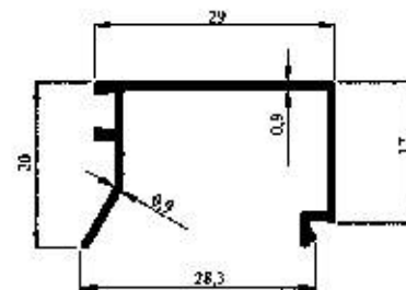
Profil No : 2124 Gramaj : 0.515 kg/m Çevre : 285 mm
