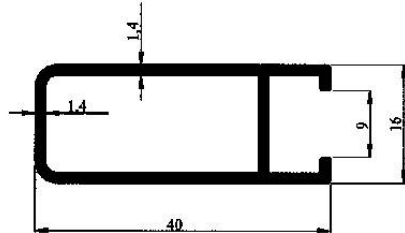
Profil No : 3222 Gramaj : 0.412 kg/m Çevre : 134 mm
