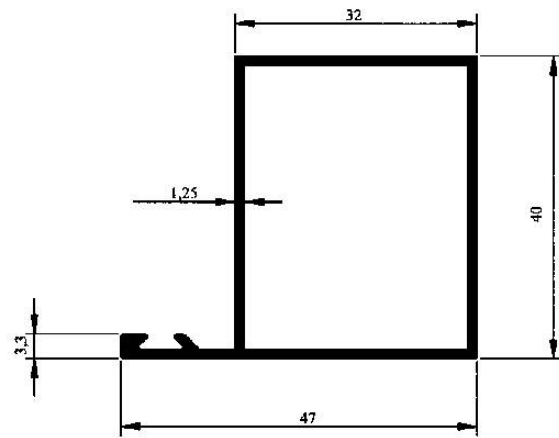
Profil No : 2602 Gramaj : 0.547 kg/m Çevre : 183 mm
