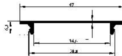
Profil No : 3881 Gramaj : 0.187 kg/m Çevre : 115 mm
