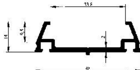
Profil No : 4013 Gramaj : 0.411 kg/m Çevre : 177 mm
