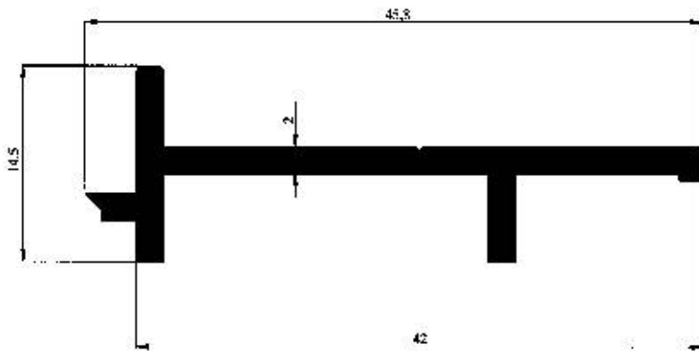
Profil No : 2411 Gramaj : 0.349 kg/m Çevre : 133 mm
