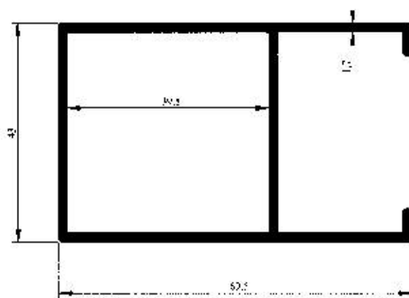
Profil No : 4019 Gramaj : 1.049 kg/m Çevre : 295 mm
