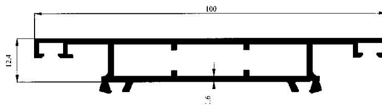
Profil No : 2547 Gramaj : 0.963 kg/m Çevre : 306 mm
