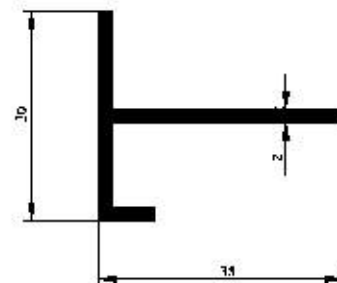
Profil No : 2041 Gramaj : 0.374 kg/m Çevre : 142 mm
