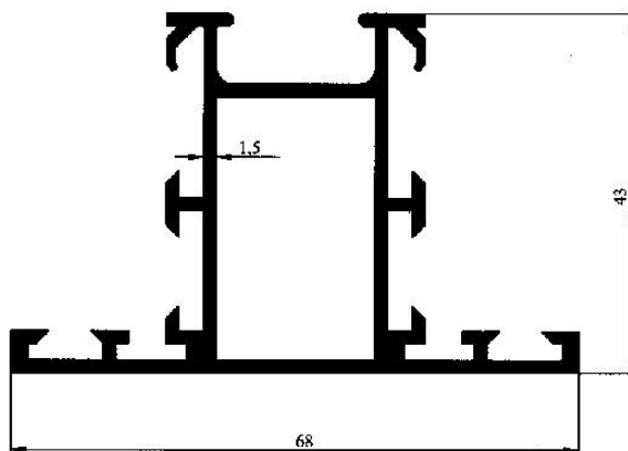
Profil No : 3211 Gramaj : 1.042 kg/m Çevre : 393 mm
