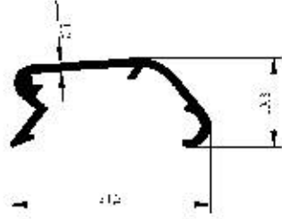
Profil No : 2895 Gramaj : 0.205 kg/m Çevre : 118 mm
