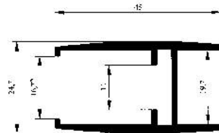
Profil No : 1958 Gramaj : 0.629 kg/m Çevre : 242 mm
