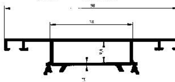
Profil No : 2352 Gramaj : 0.699 kg/m Çevre : 275 mm
