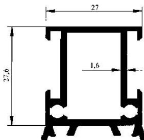
Profil No : 2539 Gramaj : 0.611 kg/m Çevre : 169 mm
