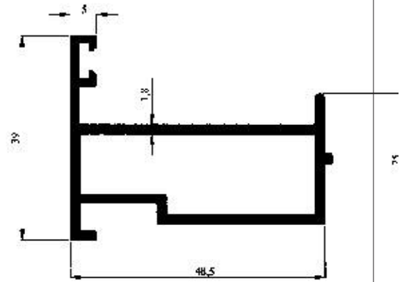
Profil No : 2438 Gramaj : 0.816 kg/m Çevre : 221 mm
