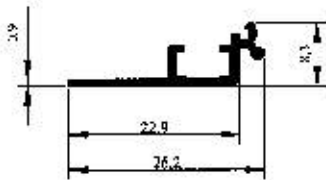
Profil No : 2798 Gramaj : 0.115 kg/m Çevre : 84 mm
