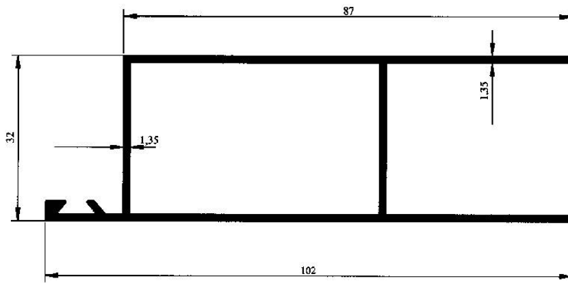
Profil No : 2618 Gramaj : 0.940 kg/m Çevre : 352 mm
