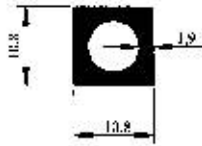
Profil No : 2256 Gramaj : 0.212 kg/m Çevre : 43 mm
