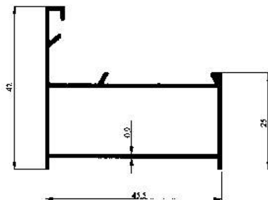
Profil No : 2127 Gramaj : 0.429 kg/m Çevre : 213 mm
