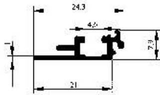
Profil No : 2742 Gramaj : 0.141 kg/m Çevre : 93 mm
