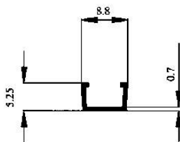
Profil No : 3097 Gramaj : 0.036 kg/m Çevre : 38 mm
