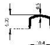
Profil No : 4729 Gramaj : 0.043 kg/m Çevre : 39 mm
