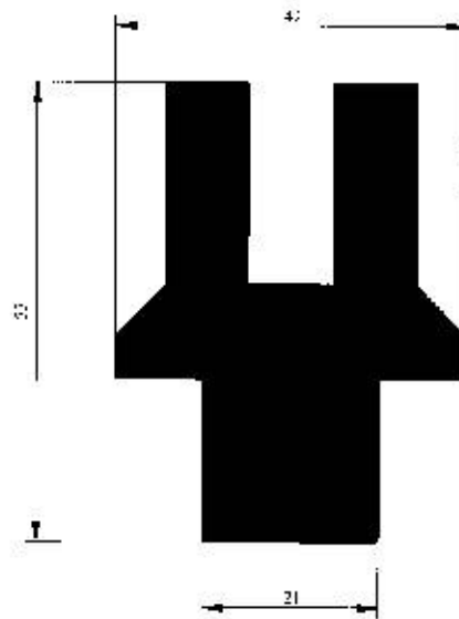
Profil No : 2226 Gramaj : 3.354 kg/m Çevre : 173 mm
