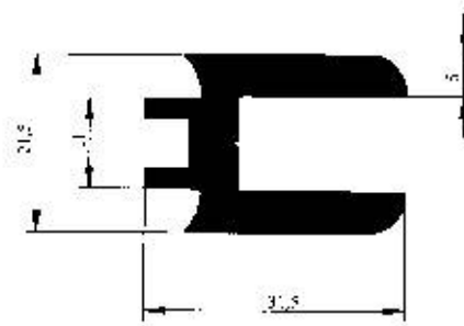
Profil No : 2229 Gramaj : 0.917 kg/m Çevre : 157 mm
