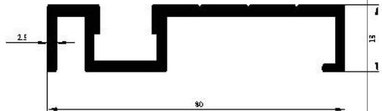
Profil No : 4730 Gramaj : 1.138 kg/m Çevre : 296 mm
