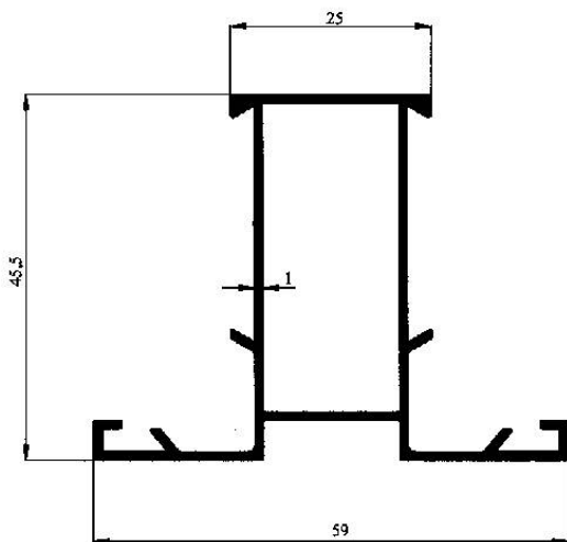
Profil No : 2101 Gramaj : 0.570 kg/m Çevre : 283 mm
