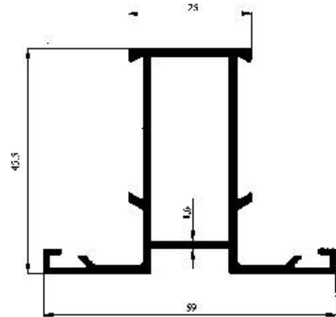
Profil No : 2150 Gramaj : 0.812 kg/m Çevre : 278 mm
