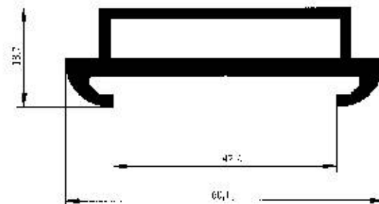
Profil No : 1974 Gramaj : 1.028 kg/m Çevre : 178 mm
