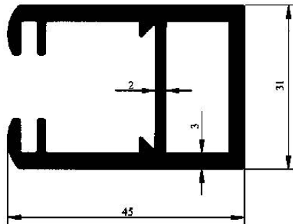
Profil No : 1901 Gramaj : 1.212 kg/m Çevre : 257 mm
