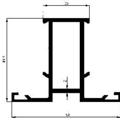
Profil No : 2151 Gramaj : 0.963 kg/m Çevre : 278 mm
