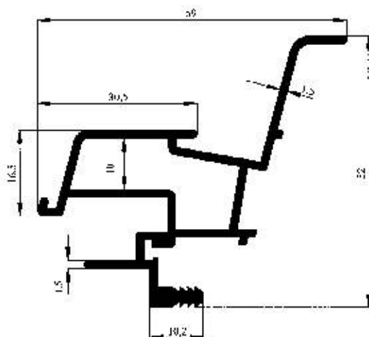
Profil No : 3071 Gramaj : 0.369 kg/m Çevre : 118 mm
