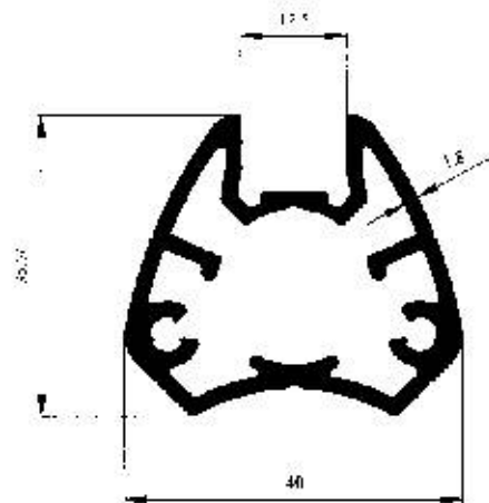
Profil No : 3031 Gramaj : 0.923 kg/m Çevre : 167 mm
