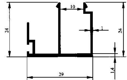
Profil No : 2944 Gramaj : 0.296 kg/m Çevre : 195 mm
