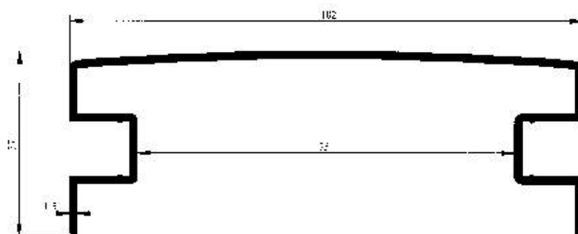
Profil No : 4004 Gramaj : 0.743 kg/m Çevre : 291 mm
