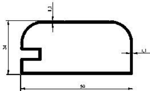
Profil No : 2123 Gramaj : 0.450 kg/m Çevre : 156 mm
