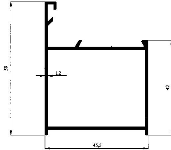
Profil No : 2085 Gramaj : 0.656 kg/m Çevre : 245 mm
