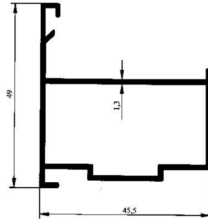
Profil No : 2030 Gramaj : 0.628 kg/m Çevre : 225 mm
