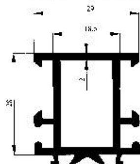
Profil No : 2351 Gramaj : 0.688 kg/m Çevre : 203 mm
