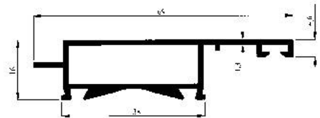
Profil No : 2453 Gramaj : 0.606 kg/m Çevre : 213 mm
