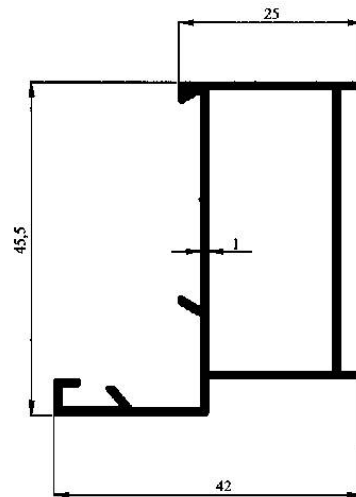
Profil No : 2085 Gramaj : 0.656 kg/m Çevre : 245 mm
