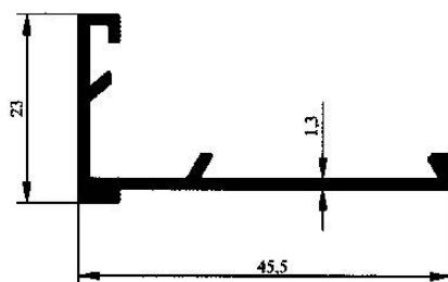
Profil No : 2026 Gramaj : 0.317 kg/m Çevre : 168 mm
