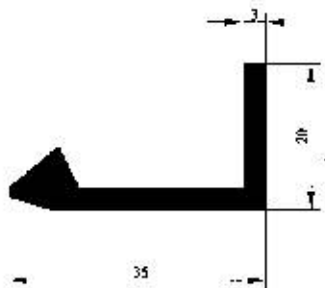
Profil No : 3860 Gramaj : 0.479 kg/m Çevre : 113 mm
