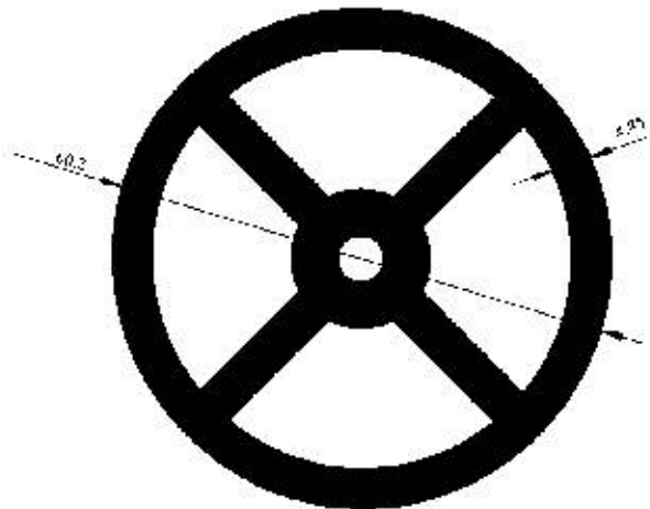
Profil No : 2230 Gramaj : 3.740 kg/m Çevre : 189 mm
