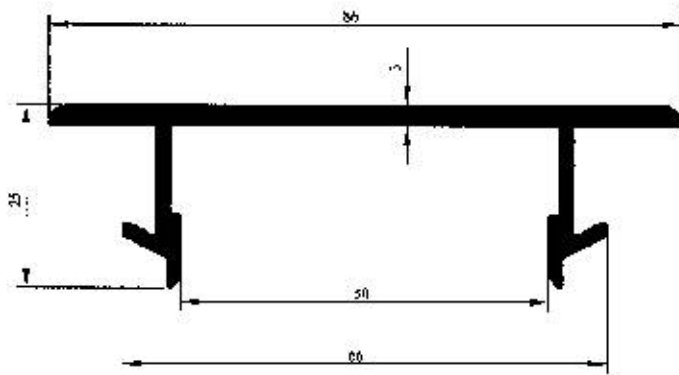
Profil No : 3835 Gramaj : 1.024 kg/m Çevre : 248 mm
