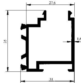
Profil No : 2545 Gramaj : 0.547 kg/m Çevre : 263 mm
