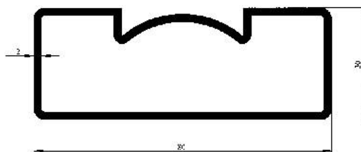
Profil No : 4726 Gramaj : 1.221 kg/m Çevre : 232 mm
