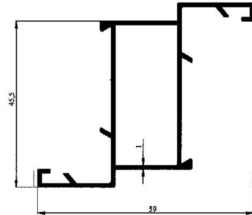
Profil No : 2100 Gramaj : 0.457 kg/m Çevre : 213 mm
