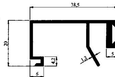
Profil No : 3210 Gramaj : 0.377 kg/m Çevre : 205 mm
