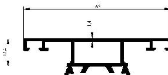
Profil No : 2348 Gramaj : 0.585 kg/m Çevre : 245 mm
