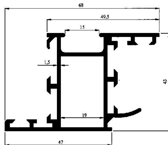
Profil No : 3212 Gramaj : 1.087 kg/m Çevre : 404 mm
