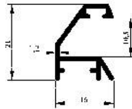
Profil No : 3110 Gramaj : 0.138 kg/m Çevre : 82 mm
