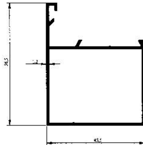
Profil No : 2040 Gramaj : 0.643 kg/m Çevre : 234 mm
