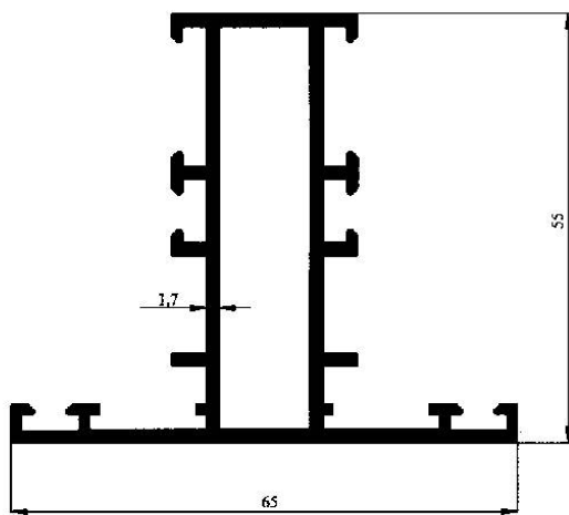
Profil No : 2512 Gramaj : 1.143 kg/m Çevre : 383 mm
