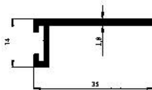
Profil No : 2042 Gramaj : 0.251 kg/m Çevre : 112 mm
